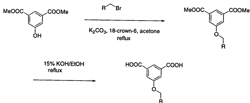
Scheme I-A
